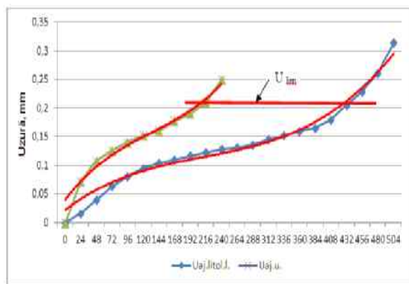
Figura 3. Evoluția uzurii ajustajului cuplelor tribologice Ø40H8/e7 testate în regim de frecare uscată și limită ungere cu LITOL:
