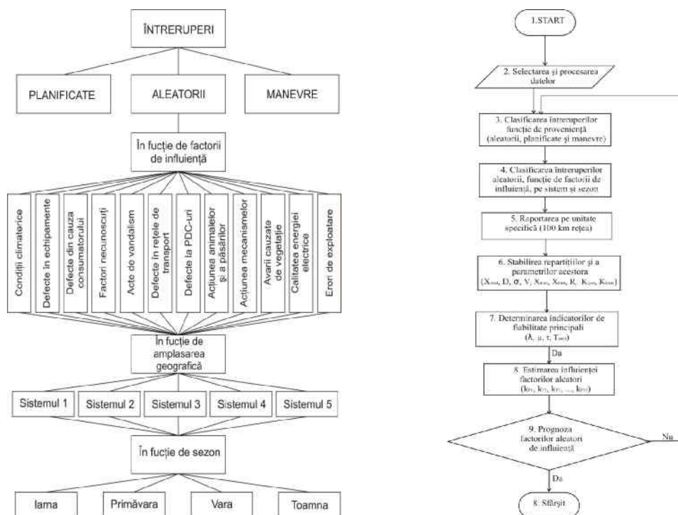
Figura 1. Schema de clasificare a întreruperilor (a), algoritmul de calcul și prognoză a fiabilității (b)
