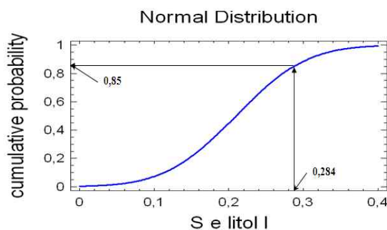
Figura 5. Probabilitatea cumulativă a datelor experimentale privind distribuția jocului efectiv în rezultatul testării tribologice a cuplelor metalopolimerice Ø40H8/e7 ungere cu LITOL 24 în regim limită
