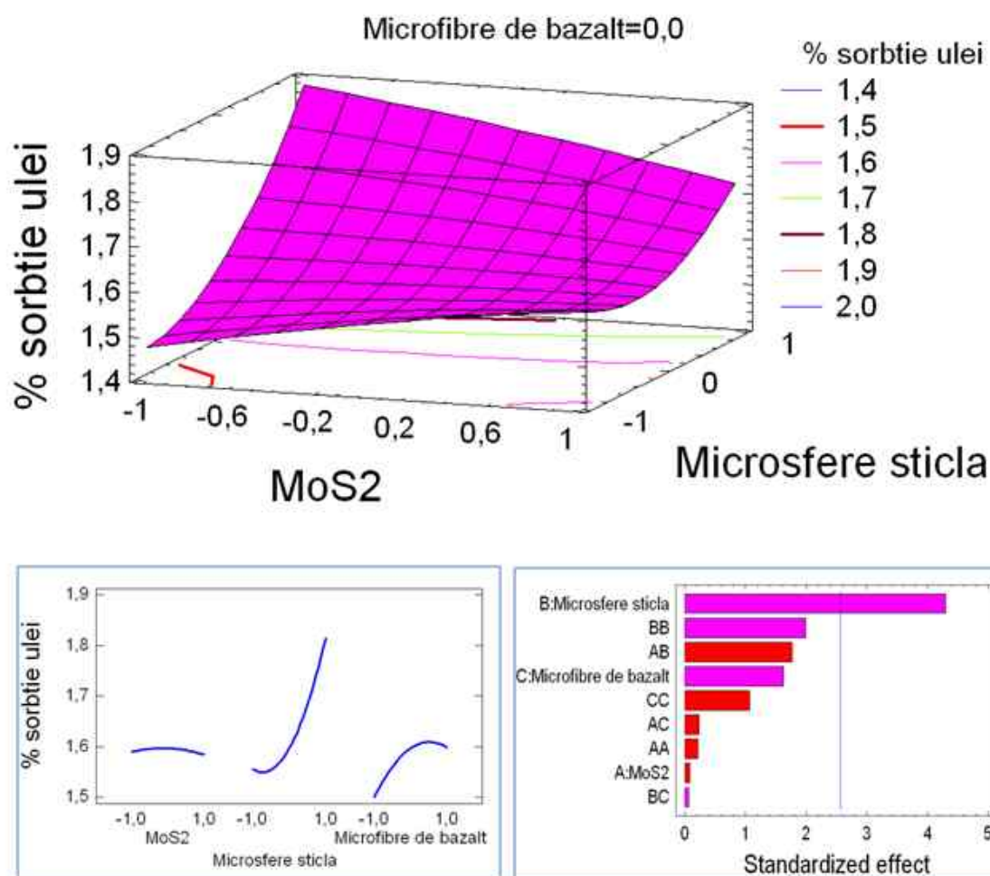
Figura 2. Prezentarea grafică a evoluției gradului de sorbție a uleiului SAE 15W40 funcție de concentrația elementelor de ranforsare
