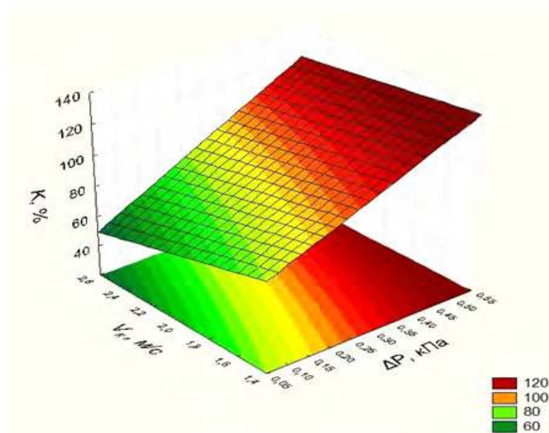
Рисунок 3. Поверхность отклика и линии равного выхода для коэффициента заполнения ячеек
