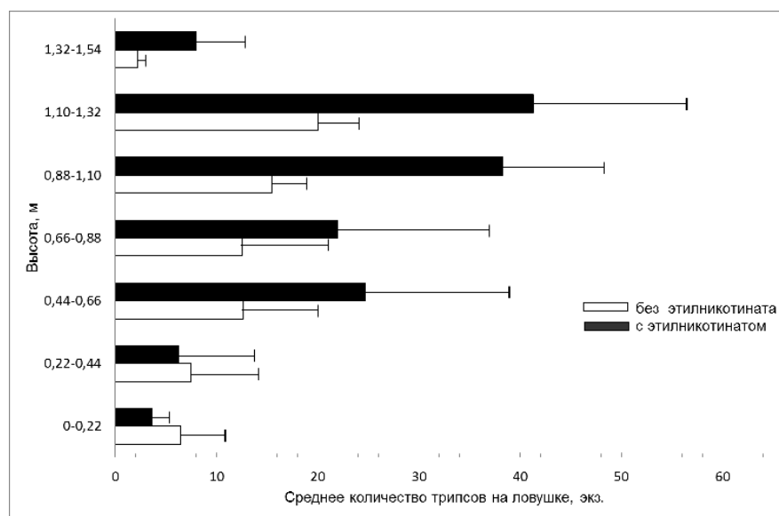
Рисунок 1. Влияние высоты ловушек на отлов табачного трипса в отсутствии и в присутствии этилникотината
