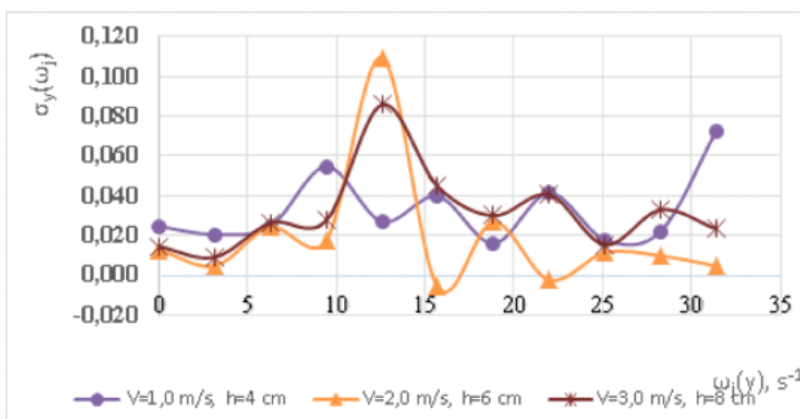
Figura 2. Reprezentarea grafică a funcției densității spectrale normate a procesului de funcționare a brăzdarului standard (pentru trei regimuri de lucru)
