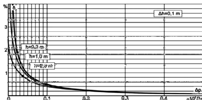
Figura 9. Eroarea de dozare \delta în funcție de suprapresiunea \Delta p din rezervorul de lucru pentru diferite înălțimi ale coloanei de lichid
