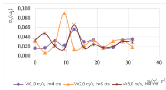
Figura 3. Reprezentarea grafică a funcției densității spectrale normale a procesului de funcționare a brăzdarului experimental cu unghiul \beta=71^\circ (pentru trei regimuri de lucru)
