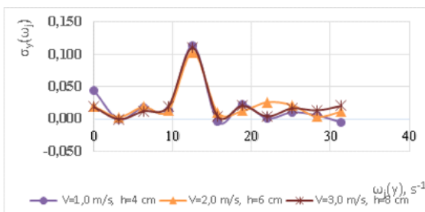
Figura 4. Reprezentarea grafică a funcției densității spectrale normale a procesului de funcționare a brăzdarului experimental cu unghiul \beta=90^\circ (pentru trei regimuri de lucru)
