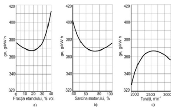
Figura 10. Efectele medii ale fracției etanolului, coeficientului de sarcină P_i/P_e și turației arborelui cotit n asupra consumului specific al motorului VAZ 2103: a) \lambda = 70\% , n = 2500 \text{ min}^{-1} ; b) C_e = 20\% \text{ vol.} , n = 2500 \text{ min}^{-1} ; c) C_e = 20\% \text{ vol.} , P_i/P_e = 70\%
