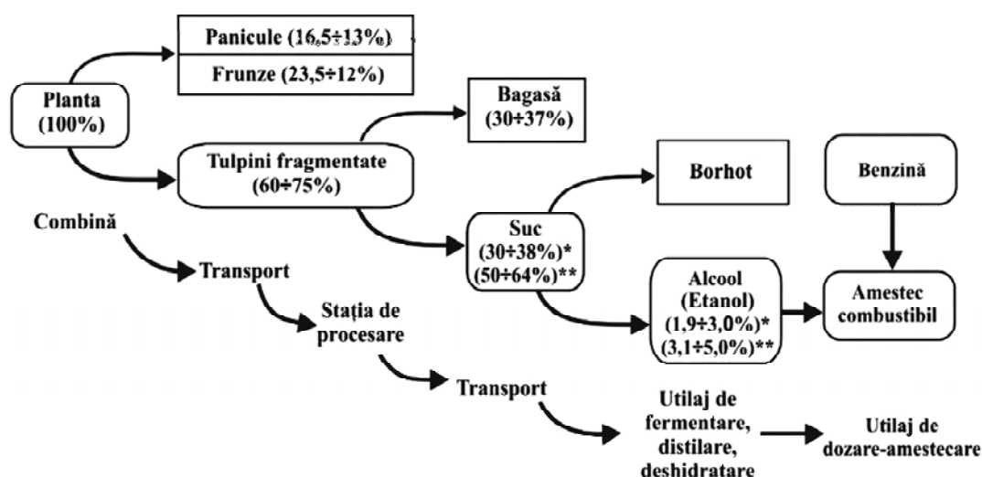
Figura 5. Schema-bloc a tehnologiei propuse pentru recoltarea și prelucrarea sorgului zaharat (cantitățile de material sunt indicate în % mas.): *presare mecanică; ** presare mecanică + imbibiție (difuzie)
