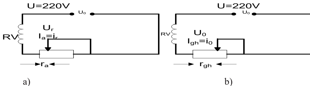
Figura 5. Schemele electrice (echivalente) ale procesului de răcire a apei (a) și formare a gheții (b): u_r , u_0 – tensiunea necesară și tensiunea sub nivel la bornele releului RV; \tau_r , \tau_0 – curentul electric necesar și curentul electric sub nivel ce asigură tensiunea necesară și tensiunea sub nivel la bornele releului RV; \tau_a = \tau_r , \tau_{gh} = r_0 – curentul electric în circuit al procesului de răcire a apei (a) și formare a gheții (b)
