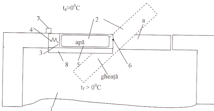
Figura 3. Gura de ventilație pentru depozitul de păstrare a fructelor și legumelor 6: 1 – depozit pentru păstrare a fructelor și legumelor; 2 – gura de ventilație; 3 – piston; 4 – arc; 5 – cameră cu volum variabil prin îngheț; 6 – ax; 7 – limitator; 8 – înveliș termoizolant; a – obturator oscilant
