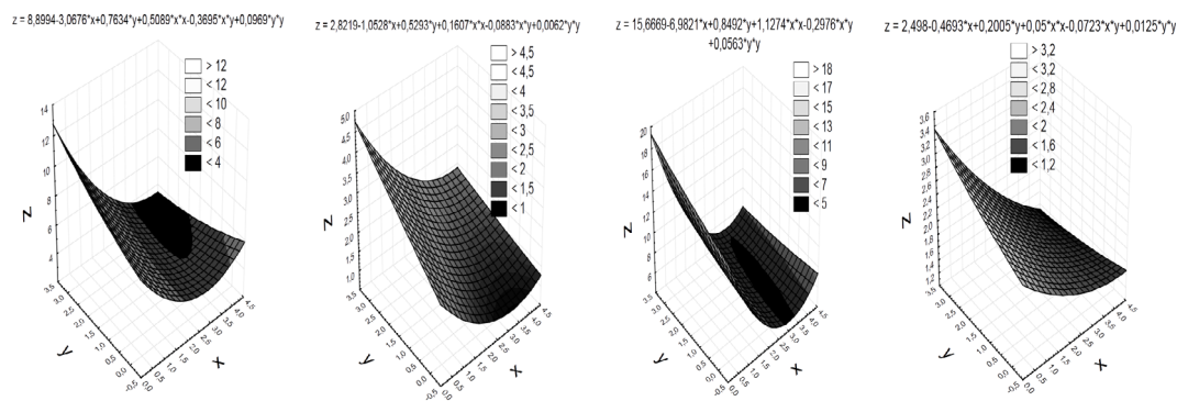
Рисунок 2. Графики зависимостей численности сорняков (ось z, шт/м²) от нормы высева (ось x, млн шт./га всхожих семян) и удобрения (ось y, в индексной форме: без удобрений – 0, N 30 P 30 K 30 – 1; N 60 P 60 K 60 – 2; N 90 P 90 K 90 – 3,0). Последовательно слева-направо и сверху-вниз: мари белая, щирица запрокинутая, щетинник сизый, пырей ползучий, бодяк полевой, среднее за 2013-2018 гг.
